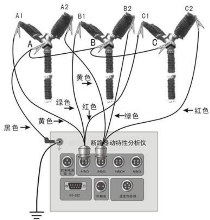
断口接线图（六断口）
